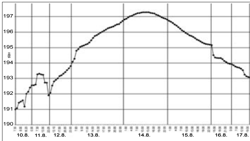
Graf závislosti nadmořské výšky hladiny, měřené na vodočetné lati u kostela v Radotíně.
